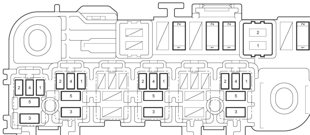
РАСПОЛОЖЕНИЕ КОНТАКТОВ ПЛАВКИХ ПРЕДОХРАНИТЕЛЕЙ И РЕЛЕ
